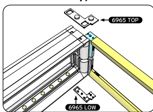
90° Type B
