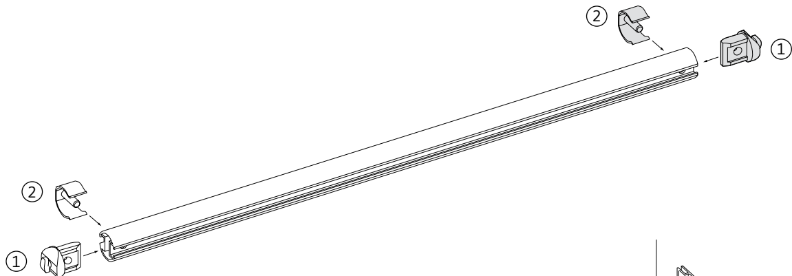
Horizontale Strebe Horizontal strut
