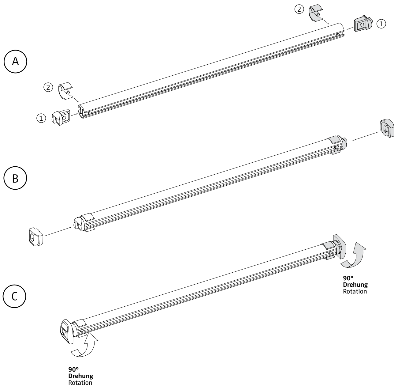
Horizontale Strebe Horizontal strut
